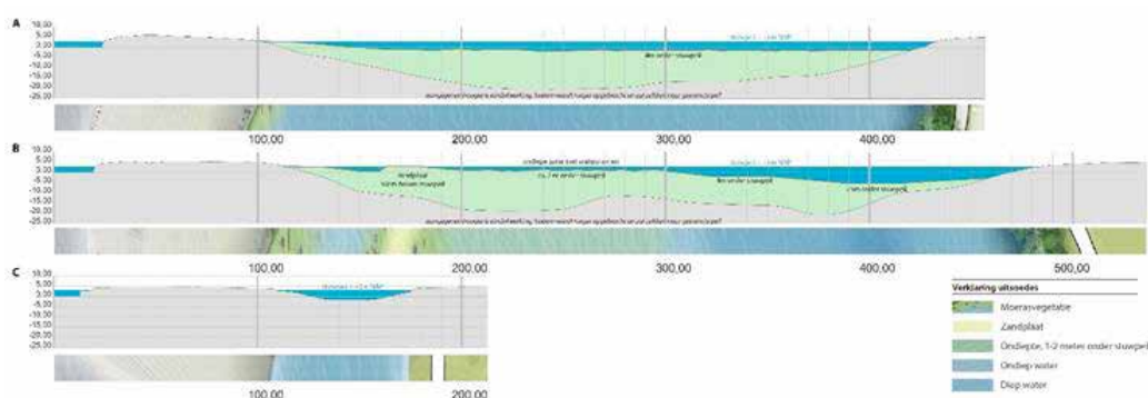
Principeschets van drie dwarsdoorsneden na opvulling van een bestaande diepe zandwinplas
